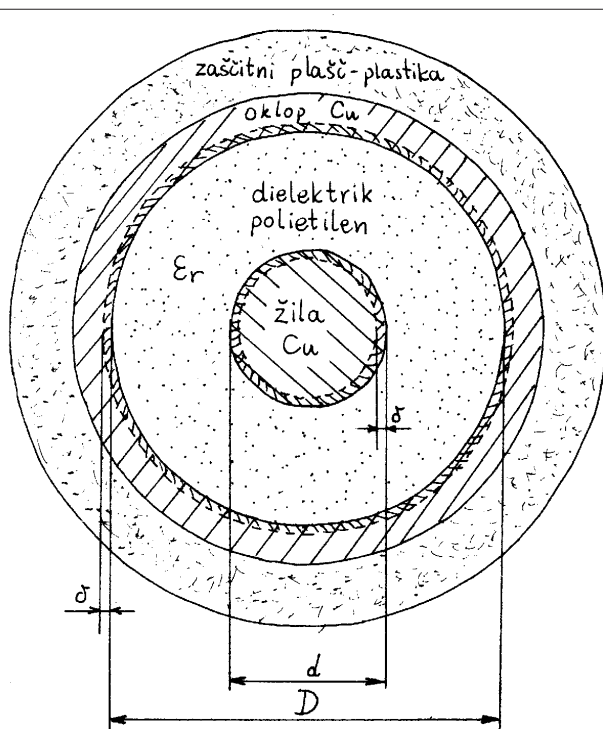
Slika 1. Prečni preseki koaksialnega kabla.
