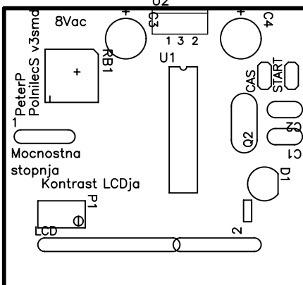
Razpored elementov zgoraj:
