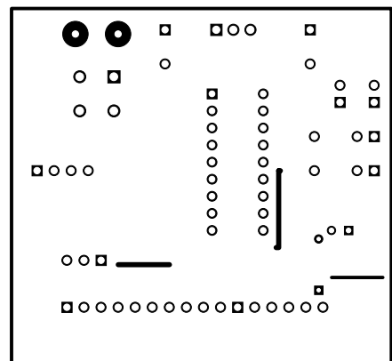
Prevezave na strani komponent (zoraj):
