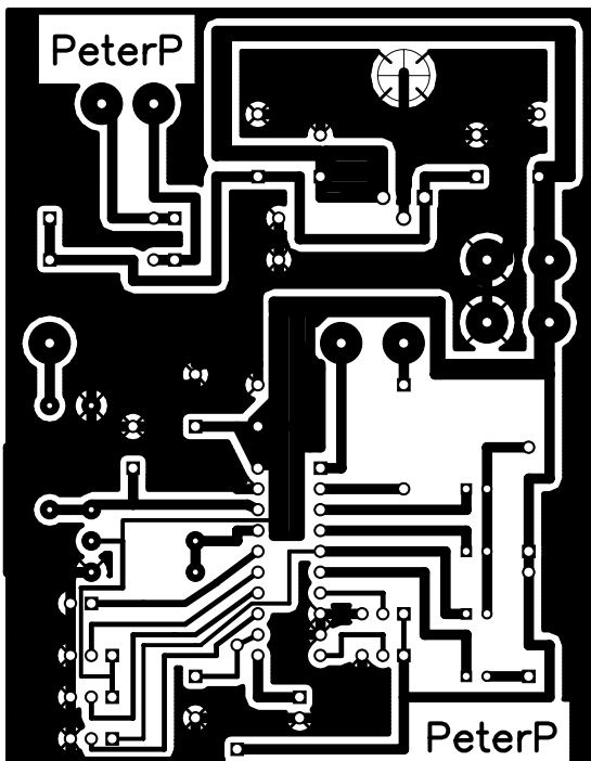
Tiskanina kontrolne stopnje:
