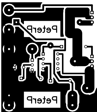
Tiskanina mocnostne stopnje:
