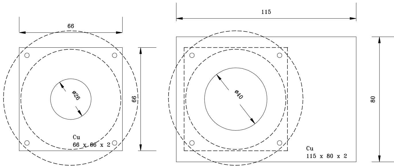
Koaksialni sklopnik
