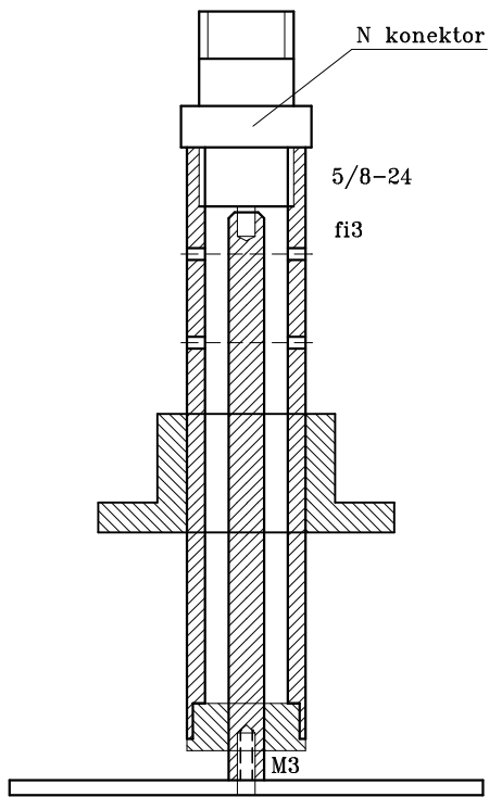
Koaksialni sklopnik
