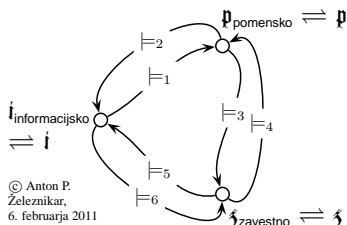
Slika 1: Polni formalistični graf informacijskega, pomenskega in zavestnega je informacijska osnova, ki ponazarja nastajanje te triade. Operatorji \models_1, \models_2, \dots, \models_6 so opisani v besedilu gesla informacijski .
